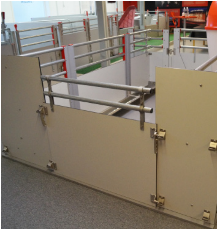
FUNKI FIBER mit Türe in voller Buchtenbreite
