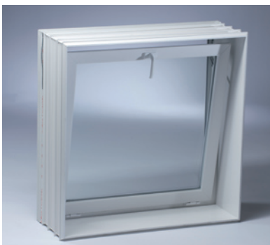
ACO Funki Kunststoff-Stallfenster Therm mit Kippflügel und Olive oben, Mauerwerk mittig
