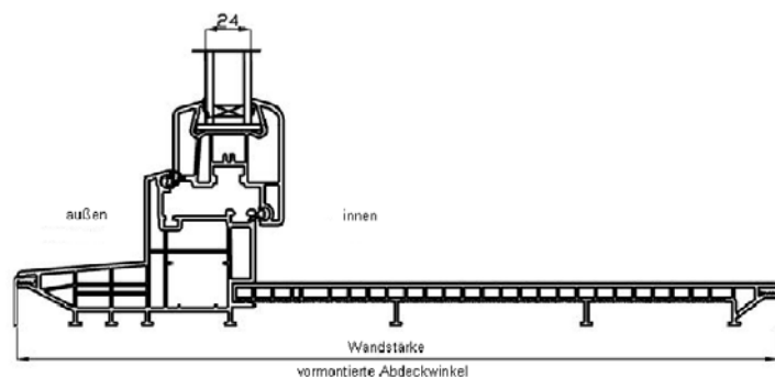
ACO Funki Kunststoff-Stallfenster Therm mit Kippflügel und Olive oben, Mauerwerk mittig
