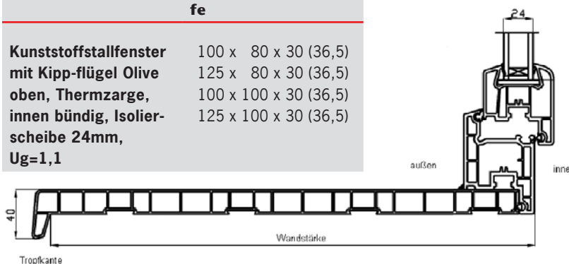
ACO Funki Kunststoff-Stallfenster Therm mit Kippflügel und Olive oben, innen bündig
